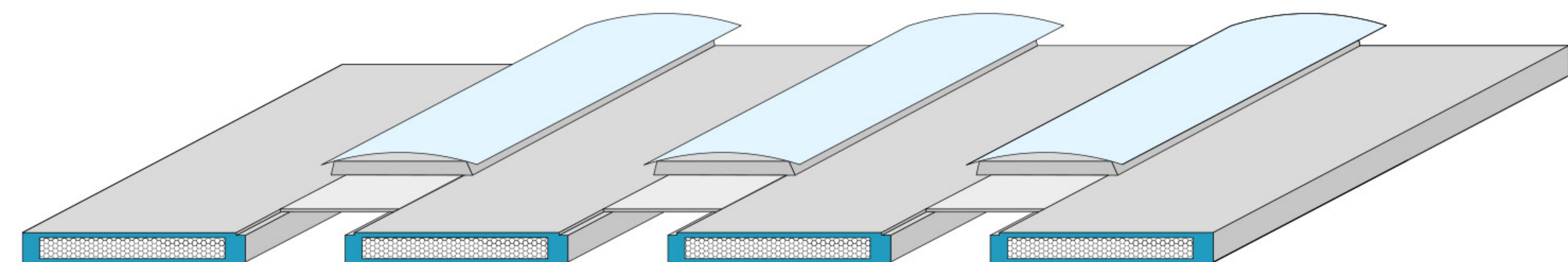
PARTICOLARE LUCERNARI DA COPERTURA
